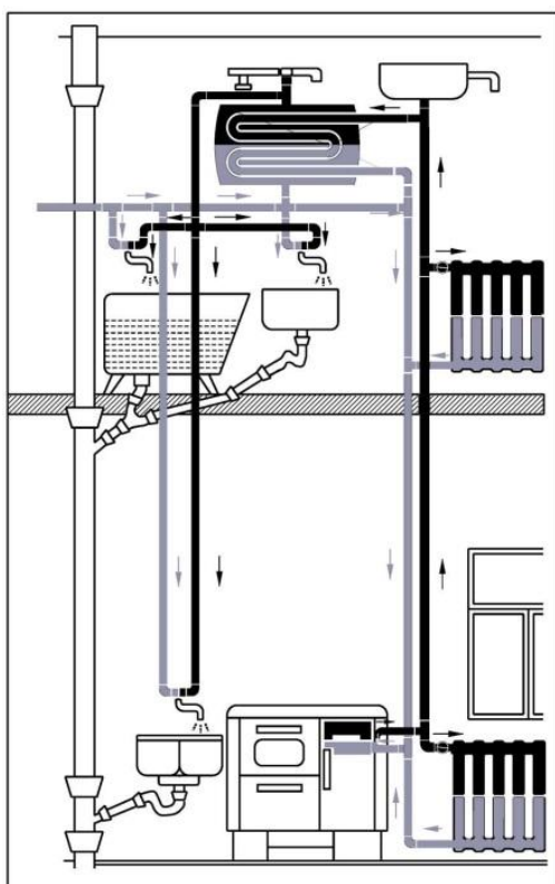
Schemat instalacji ciepłej wody w kuchni węglowej KATARZYNA
